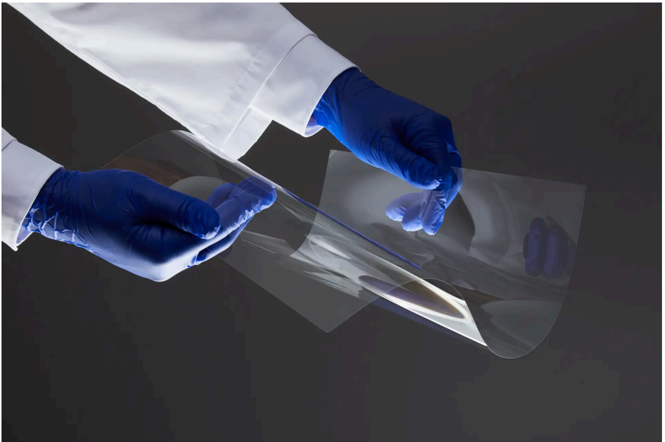
Alpair 5Gに採用された特殊ガラス 化学強化専用超薄板ガラス「Dinorex UTG®」 ガラスながら最薄0.025mm（25μm）という厚みで、直径3mm（R1.5）以下の折り曲げが可能
